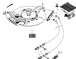
ETB-022332, Dno z otworami hydrauliczne (2)
