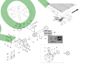
ETB-022333, Napęd mechaniczny / wałek przekąźnikowy
