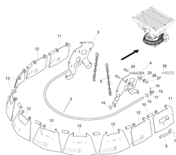
ETB-022339, Ekran rozsiewu
