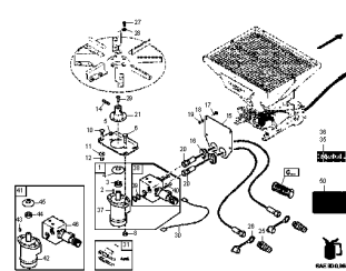
ETB-022337, Napęd hydrauliczny przez blok sterujący
