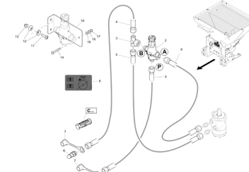
ETB-022338, Zawór regulacji przepływu
