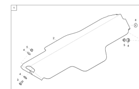
ETB-022324, Krata ochronna, uchwyt węży, osłona blaszana
