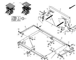
ETB-022346, Składana plandeka
