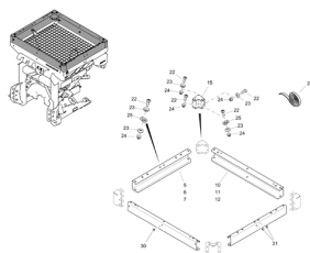
ETB-022322, Nadstawka nad zbiornik S95
