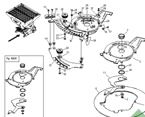
ETB-022329, Dno z otworami ręczne
