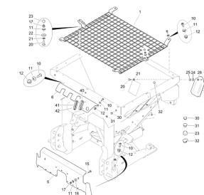
ETB-022324, Krata ochronna, uchwyt węży, osłona blaszana
