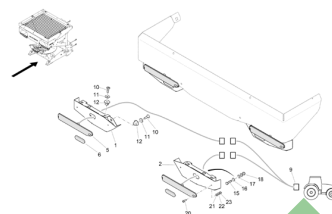
ETB-022340, Elektryczny ekran rozsiewu Easy
