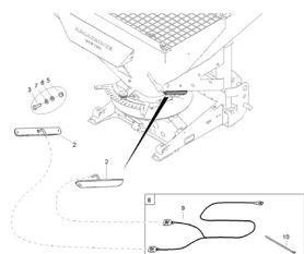
ETB-022343, Oświetlenie robocze
