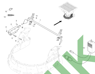
ETB-022341, Elektryczny ekran rozsiewu
