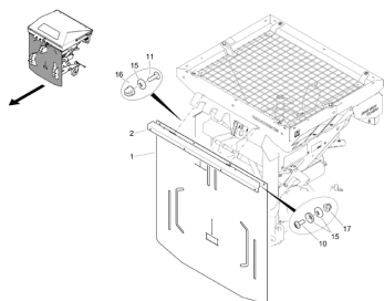
ETB-022325, Uszczelka gumowa przeciwbłotna 301
