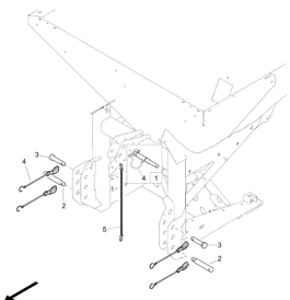
ETB-022321, Sworzeń mocujący
