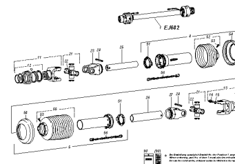
ETB-0000005689, Wałek przegubowo-teleskopowy EJ682 - W 100 E 810 mm, 1 3/8 cala, 6 sztuk
