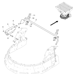
ETB-022340, Elektryczny ekran rozsiewu Easy
