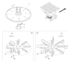
ETB-022328, Tarcza rozsiewająca i zestaw łopatek rozsiewających
