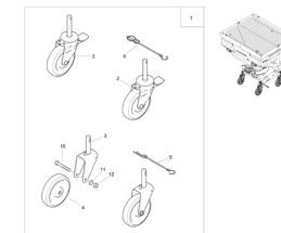
ETB-022349, Kółka transportowe, hamowane
