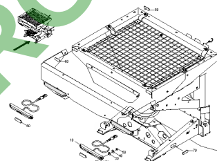
ETB-0000001249, Oświetlenie LED
