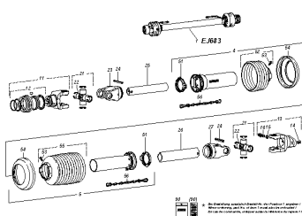
ETB-0000005841, Wałek przegubowo-teleskopowy EJ683 - W 100 E 560 mm 1 3/8 cala , 6
