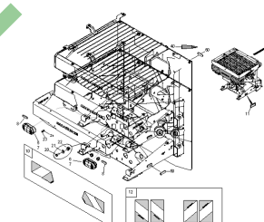
ETB-022342, Oświetlenie ze znakami ostrzegawczymi
