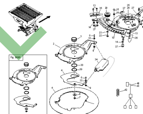
ETB-022330, Dno z otworami elektryczne
