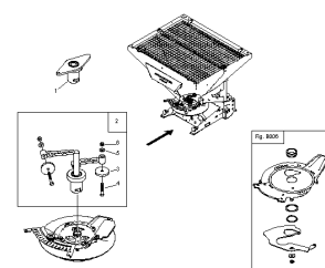
ETB-022327, Mieszadło łańcuchowe / głowica mieszająca do nawozu
